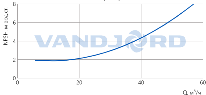
Характеристика NPSH
