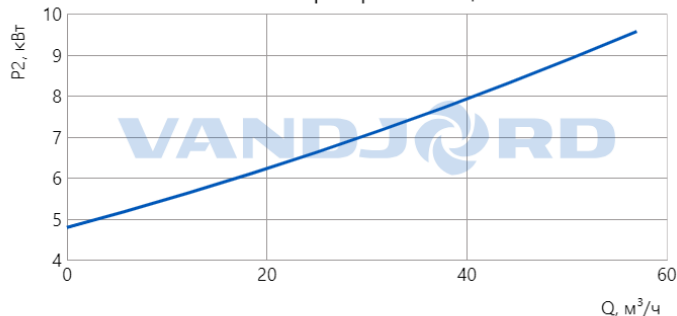
Характеристика мощности
