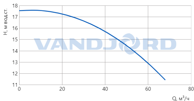
73116130 - TPV 80-150-3/2 Q-A-BT-E Гидравлическая характеристика
