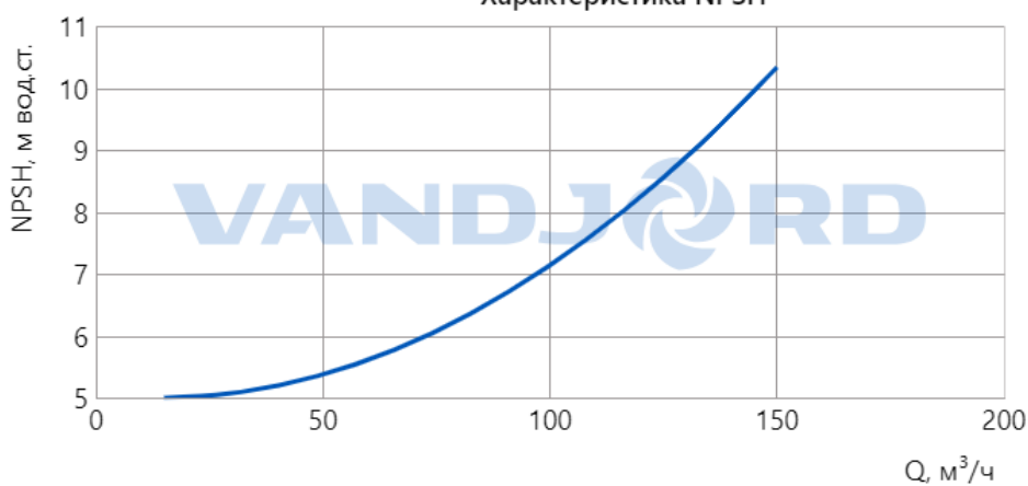
— TPV 80-910-55/2 Q-A-BT-E
