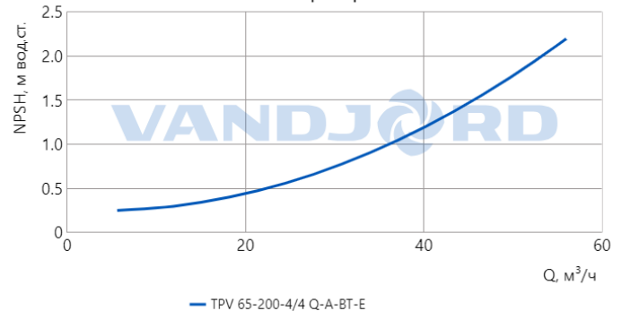
Характеристика NPSH
