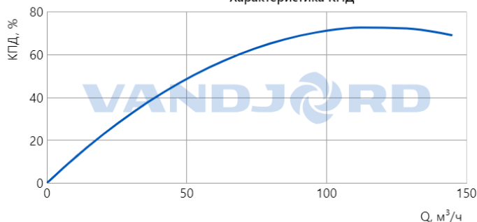
Характеристика КПД
