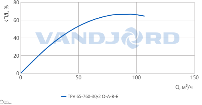
Характеристика КПД
