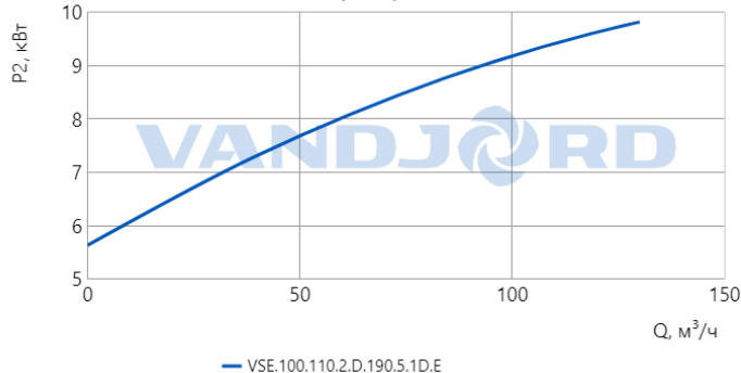
Характеристика мощности
