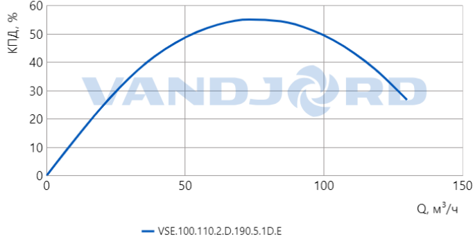
Характеристика КПД
