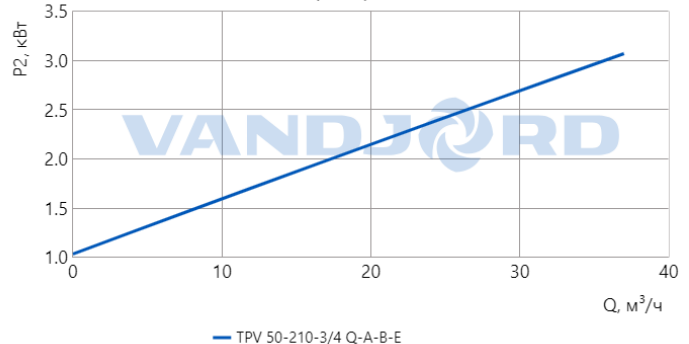
Характеристика мощности
