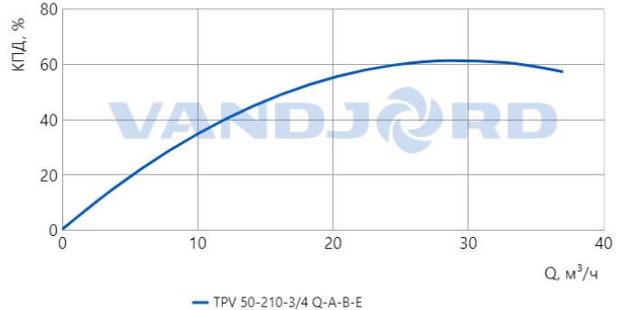
Характеристика КПД
