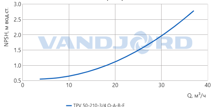
Характеристика NPSH
